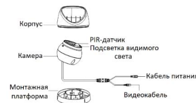
Рисунок 1-18 Камера «шар» III типа
